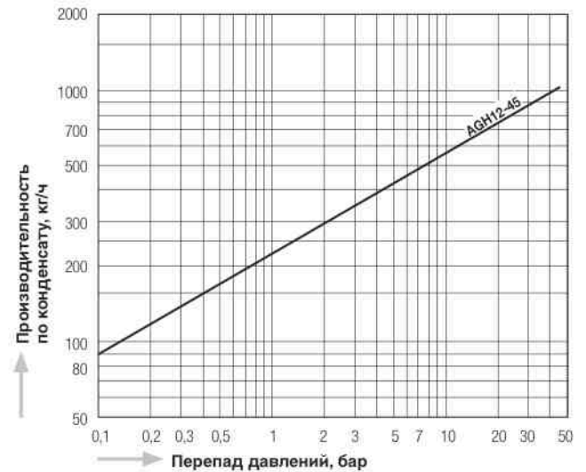
График производительности AGH12-45
